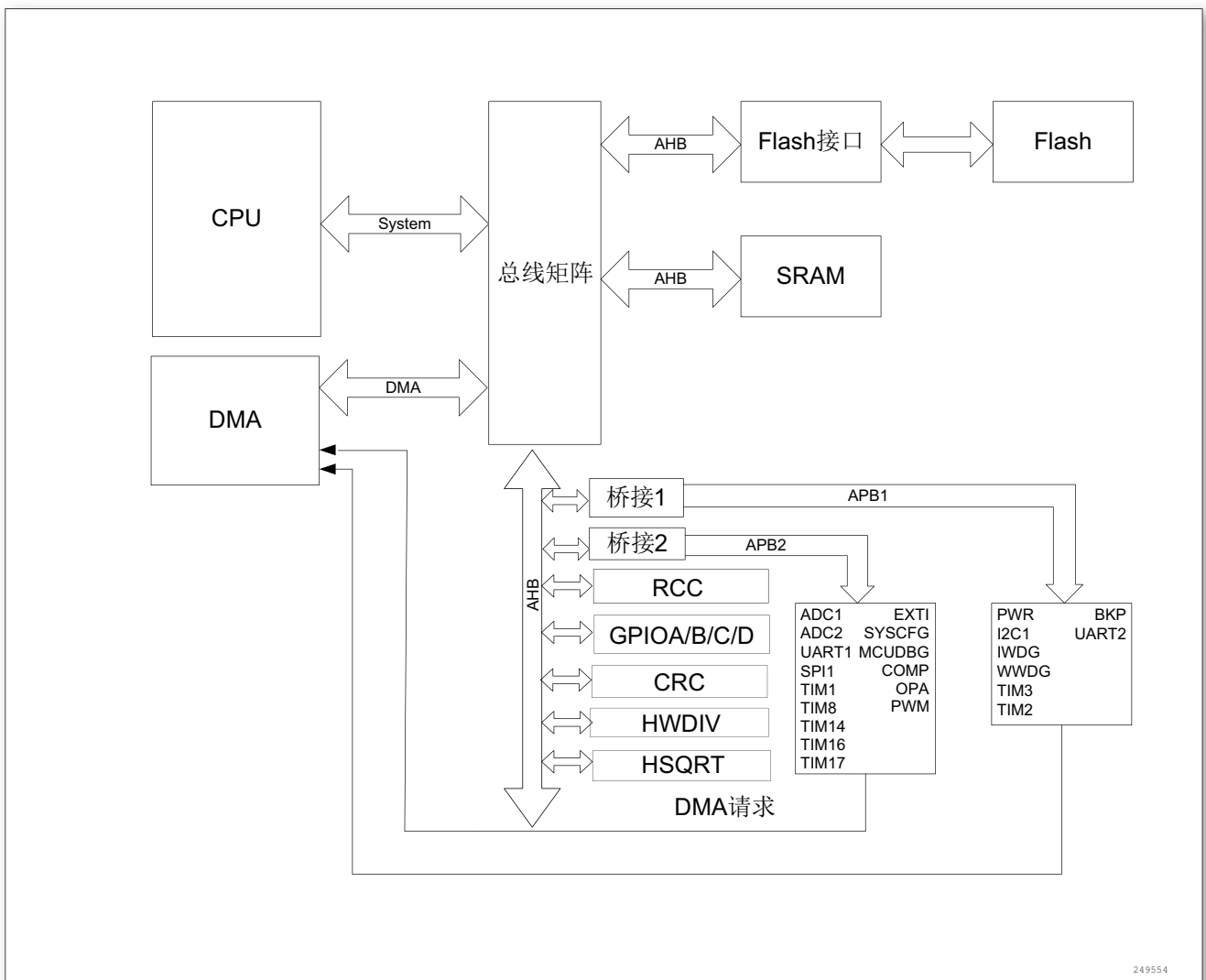
图 1. 模块框图
